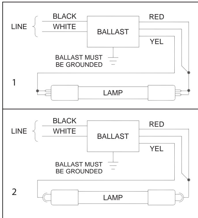
Wiring Diagrams
